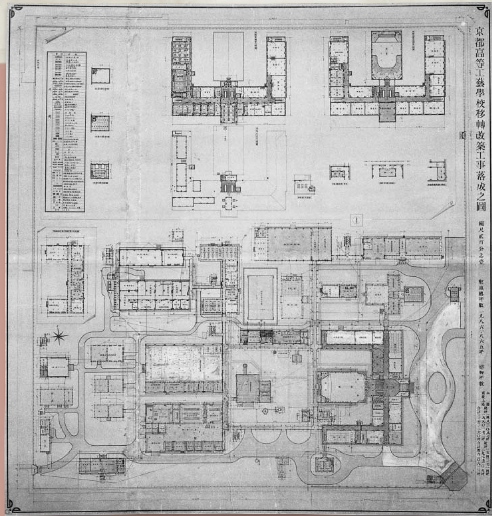
京都高等工芸学校移転改築工事落成元図
